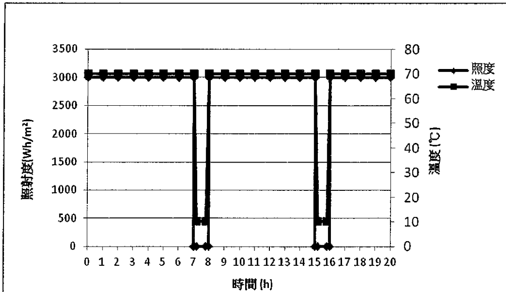
圖 1. 溫度及輻射照度循環
